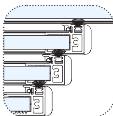
Montante rinforzo anta > profilo di rinforzo montante anta con funzione anche di antispiffero
