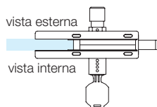
APERTURA INVERSA serratura chiave interna maniglia esterna, vista interna.
