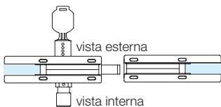
APERTURA DI SERIE serratura chiave esterna maniglia interna, vista interna.
