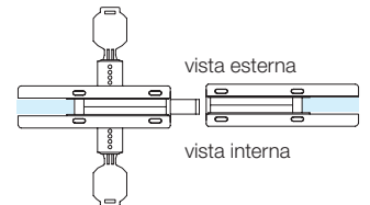
APERTURA INVERSA serratura con chiave esterna/interna, vista interna.
