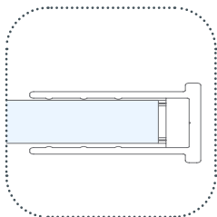
Profilo laterale > profilo in alluminio laterale di compensazione e finitura
