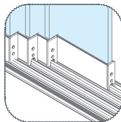
Guida inferiore > guida di scorrimento inferiore con carrelli in acciaio inox e cuscinetti a sfera, per un movimento fluido e silenzioso
