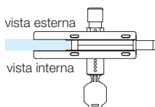
APERTURA INVERSA serratura chiave interna maniglia esterna, vista interna.
